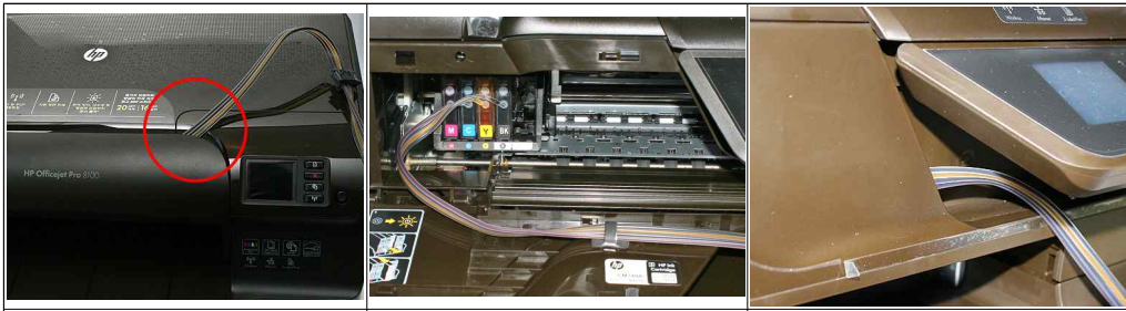
신형 그림 1-13 이제 뒷덮개를 닫고 정면덮개를 닫을 때 케이블을 사진처럼 정리해주세요. 전원이 켜져 있으면 내부에 카트리지 이동이 시작합니다. 신형 그림 1-14 HP8600의 경우 그림처럼 덮개의 스티커 바로 뒷 부분에 부착해주세요. 나머지는 8100과 같습니다. 신형 그림 1-15 HP8600은 덮개를 닫았을 때 그림처럼 잉크호스가 빠져주면 정상설치된 것입니다.
